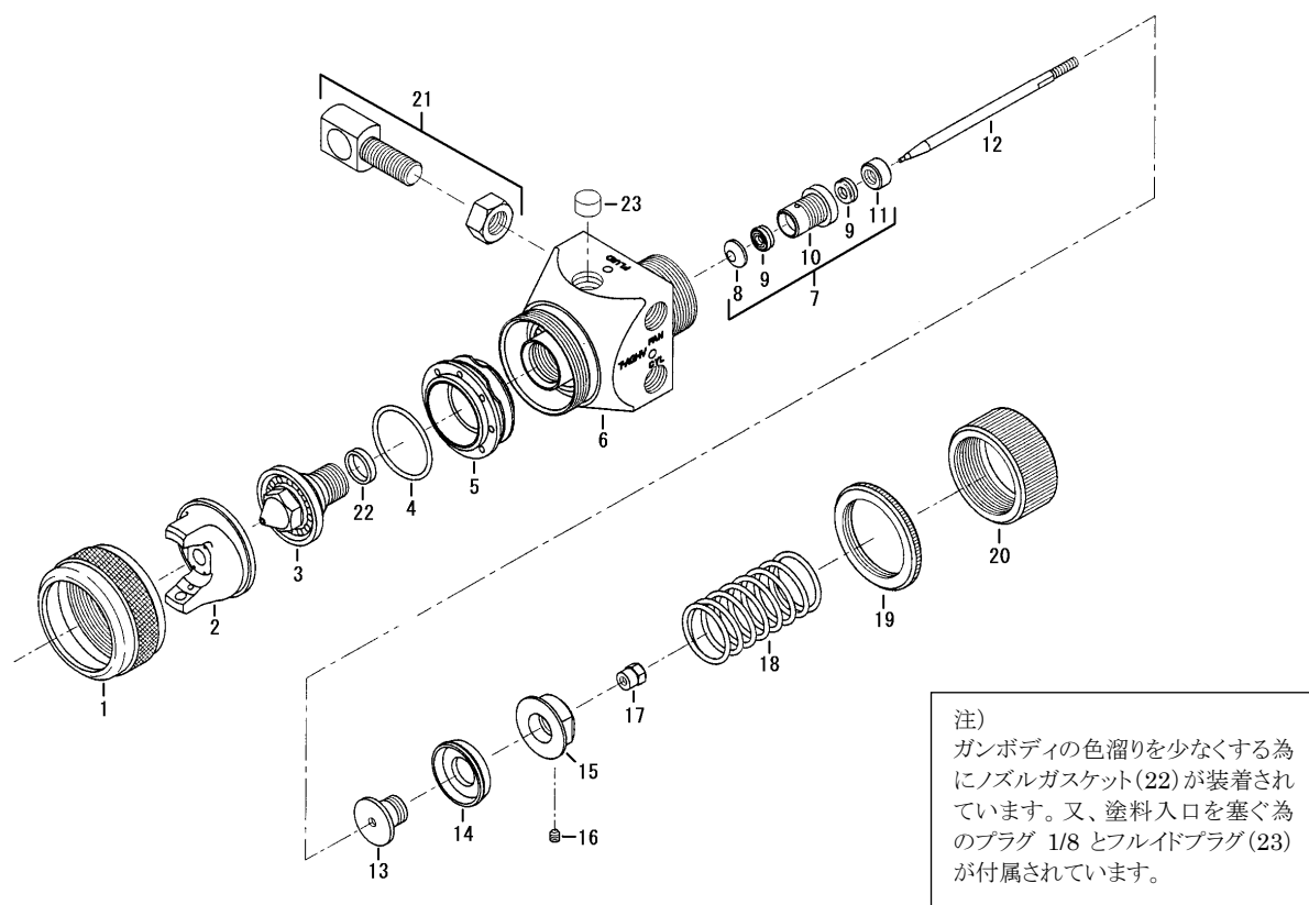
図. 5 ガン分解図
